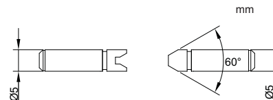
Rosca ângulo 60°
